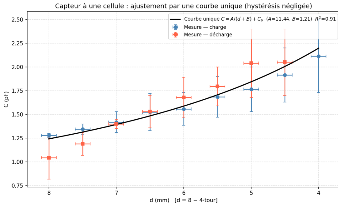
Figure 10. Capteur à une cellule unique : capacité mesurée (deux essais moyennés, branches de charge et de décharge) en fonction de d = 8 - 4 tour, ajustée par une unique courbe C = A/(d + B) + C_b . Les barres d'erreur, très larges, traduisent le caractère improvisé du montage ; les points de charge et de décharge se confondent en leur sein.
