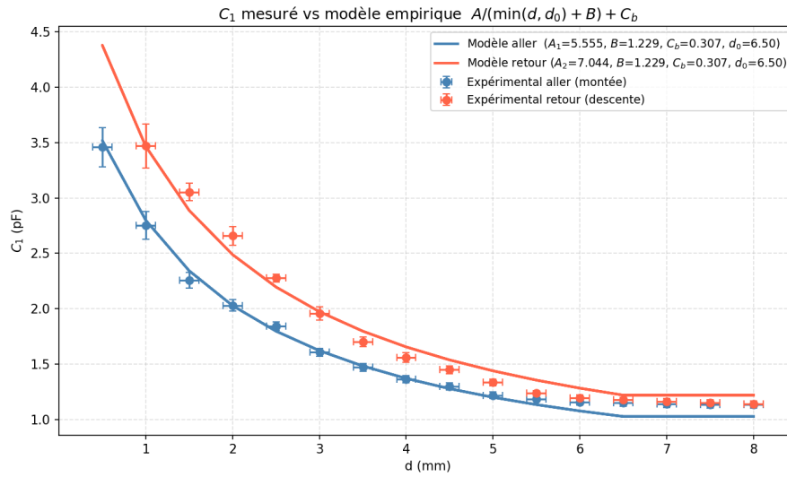
Figure 8. C_1 en fonction de d . Avec le fit, on pose \min(d, d_0) car la compression ne démarre pas à 8 mais au moment où la mousse s'écrase, c'est-à-dire d = 6,5 .
