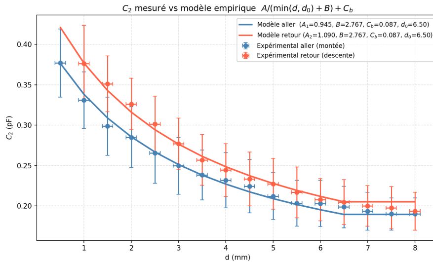
Figure 9. C_2 en fonction de d .
