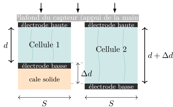
Figure 2. Premier prototype (V1) : deux cellules côte à côte, partageant le même diélectrique en mousse ( \varepsilon ) et la même surface S . Les armatures hautes sont alignées ; une cale solide surélève l'armature basse de la cellule 1, créant un décalage \Delta d , de sorte que la cellule 1 a l'écartement d et la cellule 2 l'écartement d + \Delta d . Comme \varepsilon et S sont communs, ils s'éliminent dans le rapport C_1/C_2 .
