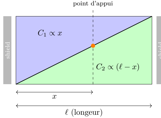
Figure 11. Capteur de position à deux triangles capacitifs complémentaires, avec blindage latéral. La surface de C_1 croît avec x , celle de C_2 décroît.
